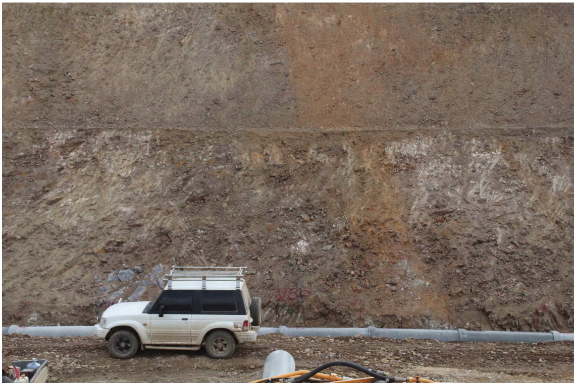
STA.1+750 하단부
