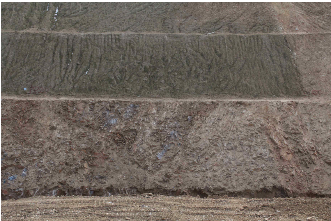
STA.1+910 하단부
